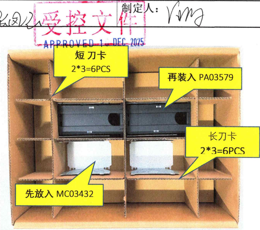
图二, 箱子底部先装一个隔板, 再将刀卡装好放入箱子, 1 层 8 格, 1 格装 1 个 PA03579+MC03432, 装满后盖上隔板, 一箱 2 层, 共 16 个。
